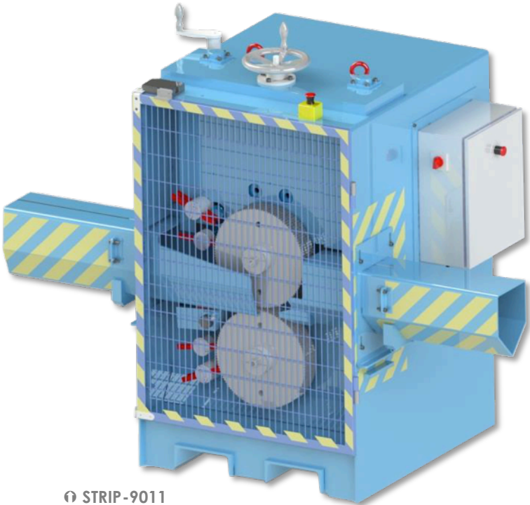
STRIP-9011 Dénudeur grande capacité : câbles Ø 10 à 160 mm
