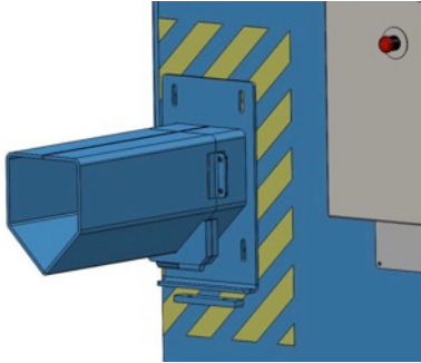
STRIP-9011 Dénudeur grande capacité : câbles Ø 10 à 160 mm
