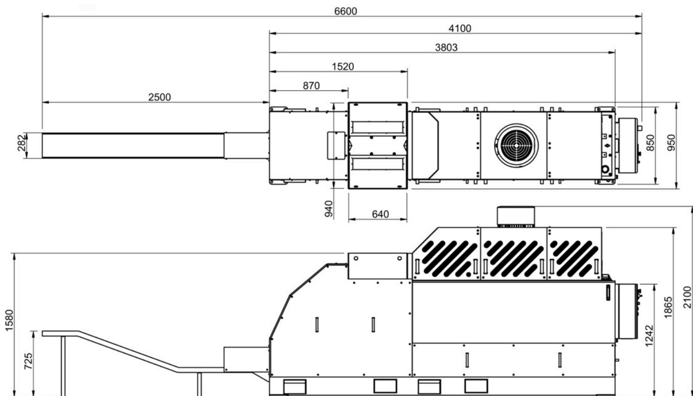
ⓘ METALLICAN-M40 Dimensions en millimètres
