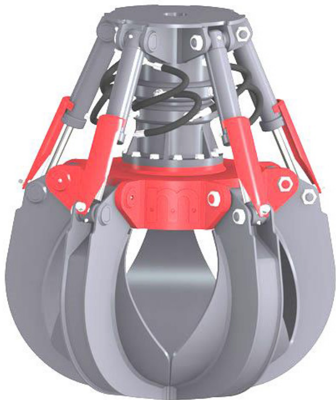
Combiné Grappin & Plateau magnétique STAR-MAGNET
